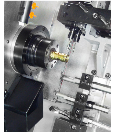
Furar e rosquear transversal
