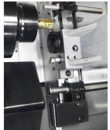
Tornear polígonos e fresar rosca
